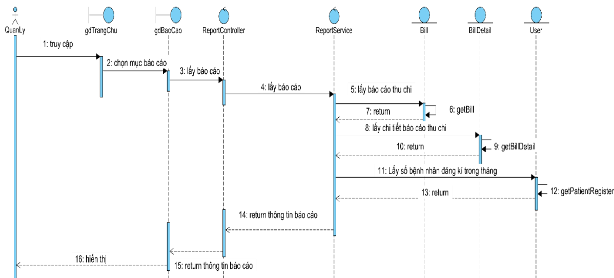
Hình 2.33: Biểu đồ tuần tự chức năng báo cáo
