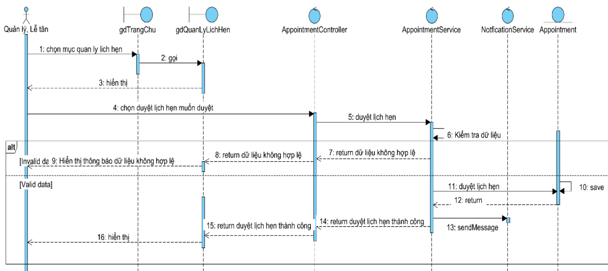
Hình 2.27: Biểu đồ tuần tự chức năng duyệt lịch hẹn
