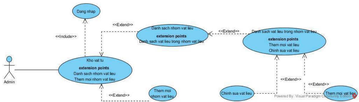
Hình 2.10: Biểu đồ use case chức năng quản lý kho vật tư
