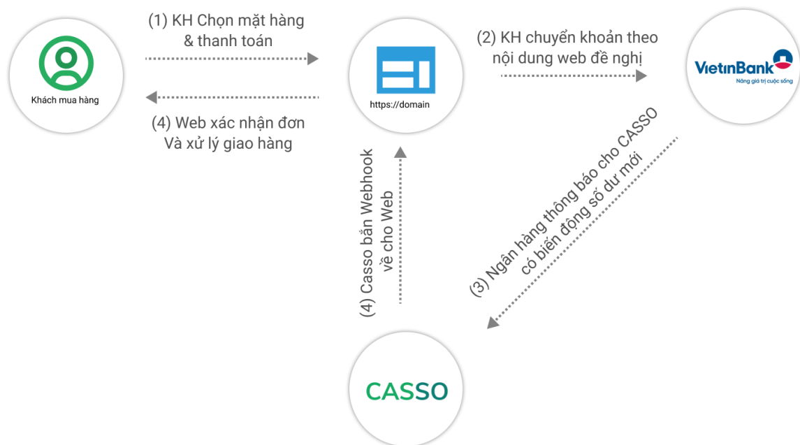
Hình 3.20: Luồng xử lý sự kiện webhook thanh toán CASSO
