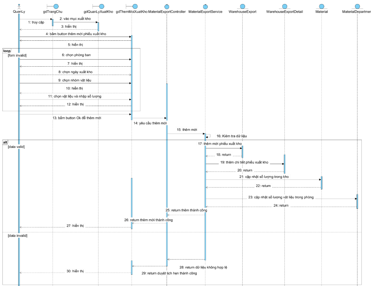
Hình 2.32: Biểu đồ tuần tự chức năng thêm phiếu xuất kho
