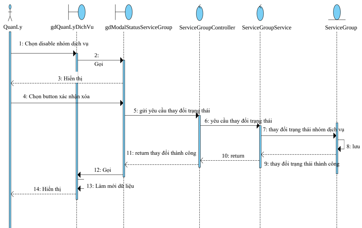
Hình 2.22: Biểu đồ tuần tự chức năng thay đổi trạng thái nhóm dịch vụ
