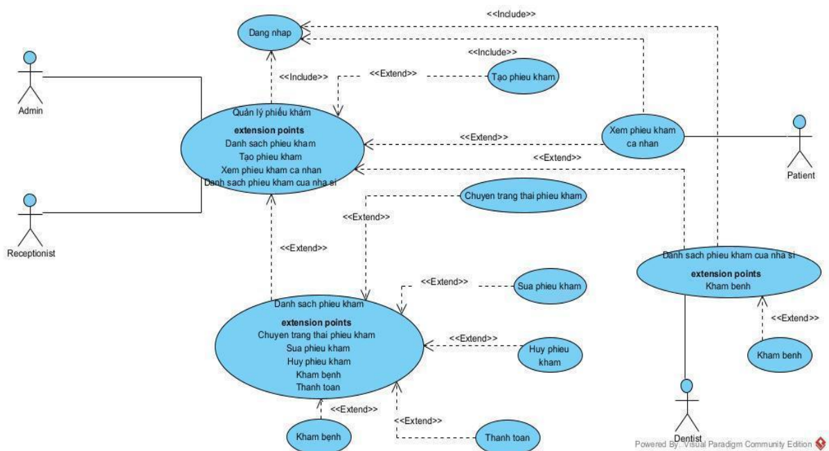
Hình 2.5: Biểu đồ use case chức năng quản lý phiếu khám
