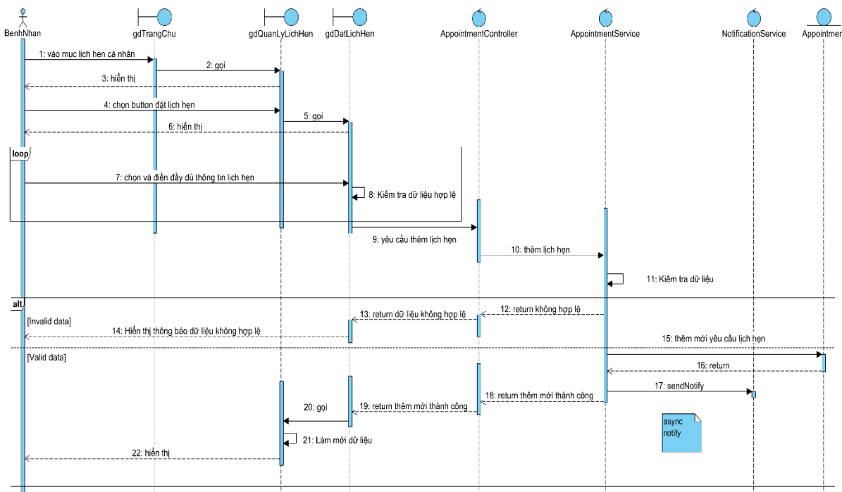
Hình 2.26: Biểu đồ tuần tự chức năng đặt lịch hẹn cho bệnh nhân
