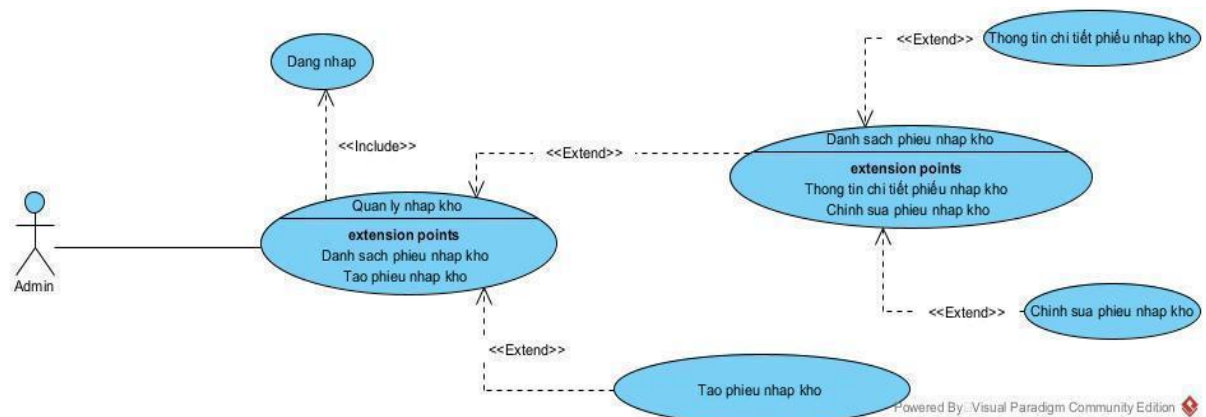
Hình 2.11: Biểu đồ use case chức năng quản lý nhập vật liệu
