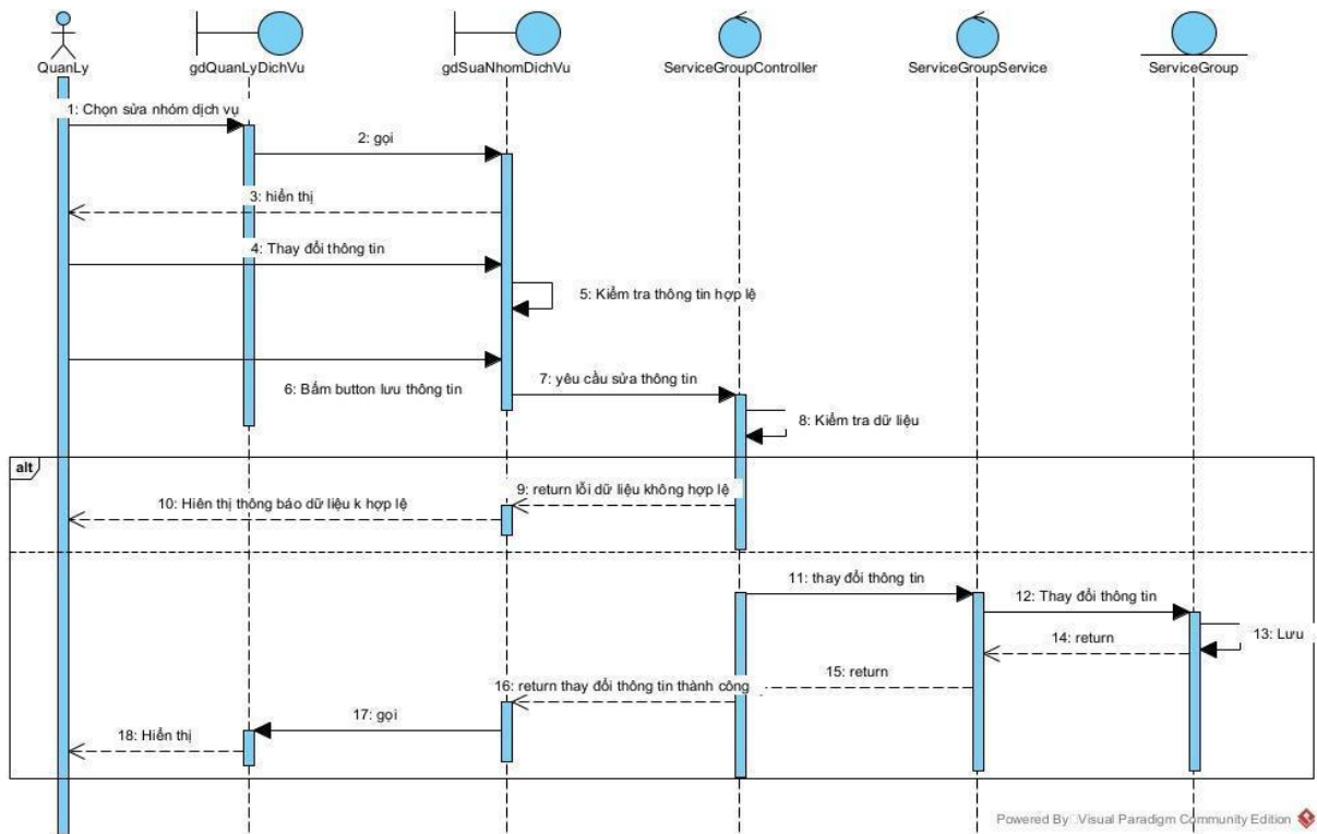
Hình 2.21: Biểu đồ tuần tự chức năng chỉnh sửa nhóm dịch vụ
