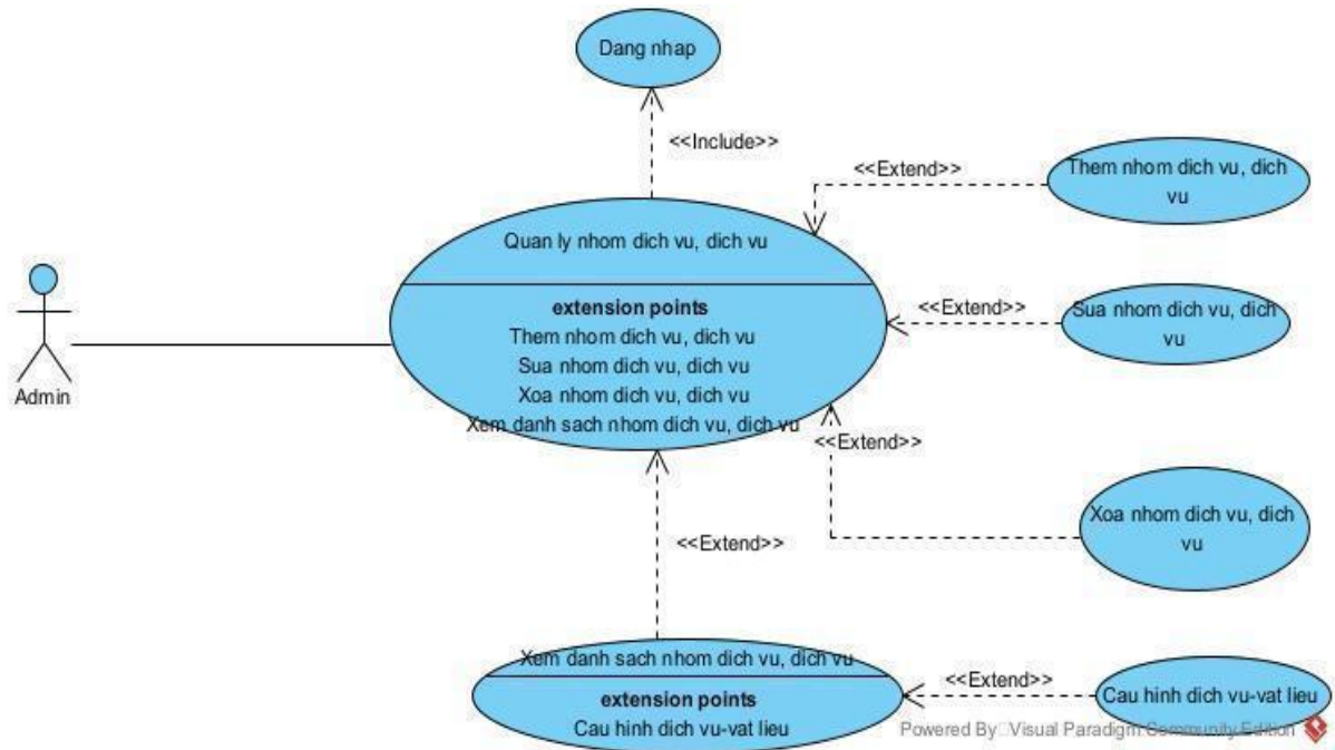
Hình 2.2: Biểu đồ use case chức năng quản lý dịch vụ
