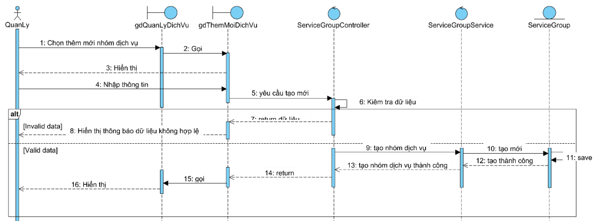
Hình 2.20: Biểu đồ tuần tự chức năng thêm nhóm dịch vụ
