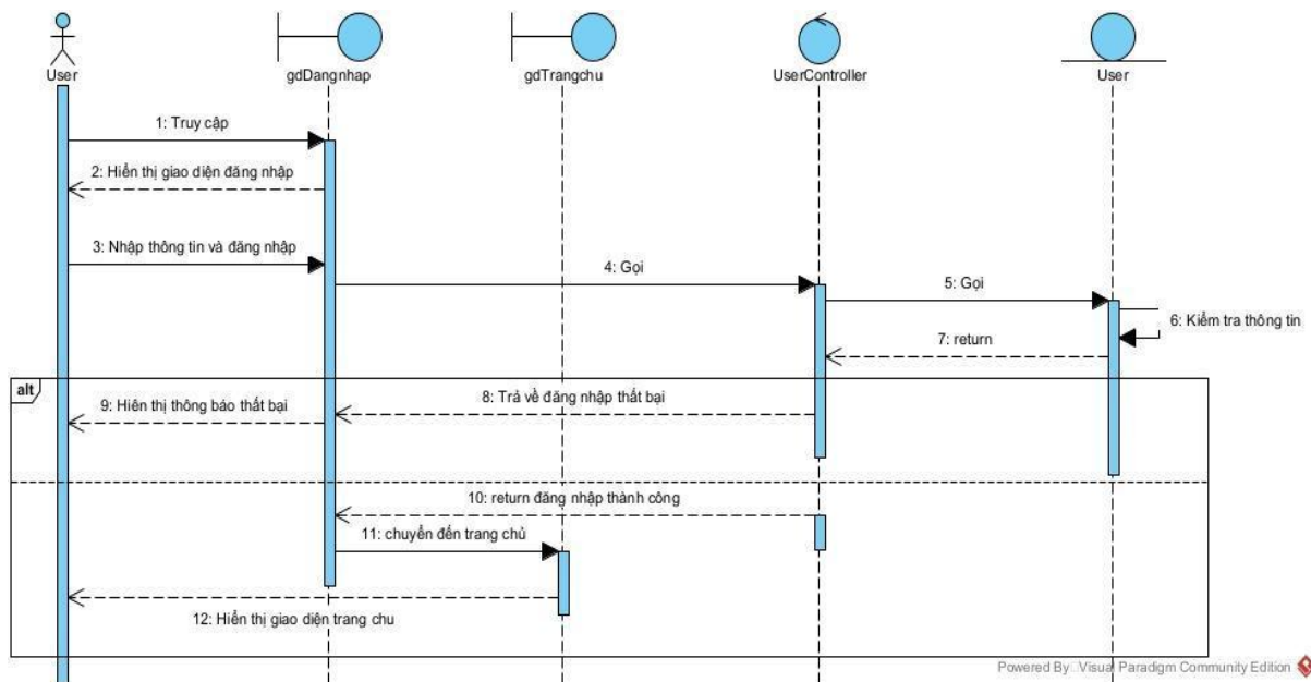
Hình 2.18: Biểu đồ tuần tự chức năng đăng nhập
