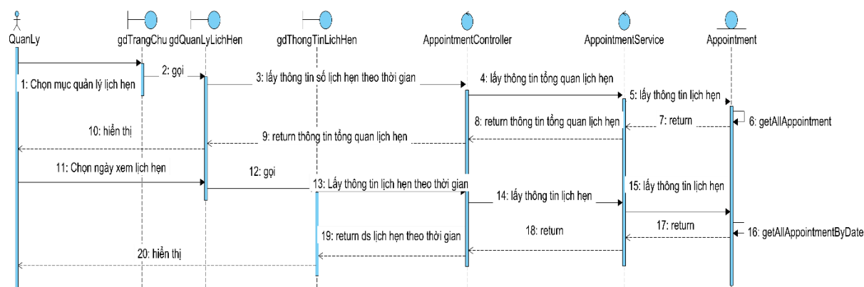
Hình 2.24: Biểu đồ tuần tự chức năng xem danh sách lịch hẹn quản lý
