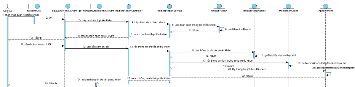
Hình 2.28: Biểu đồ tuần tự chức năng xem chi tiết phiếu khám
