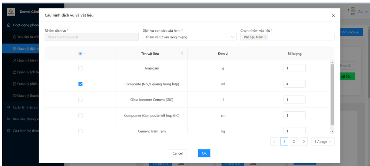
Hình 3.2: Giao cấu hình dịch vụ - vật liệu
