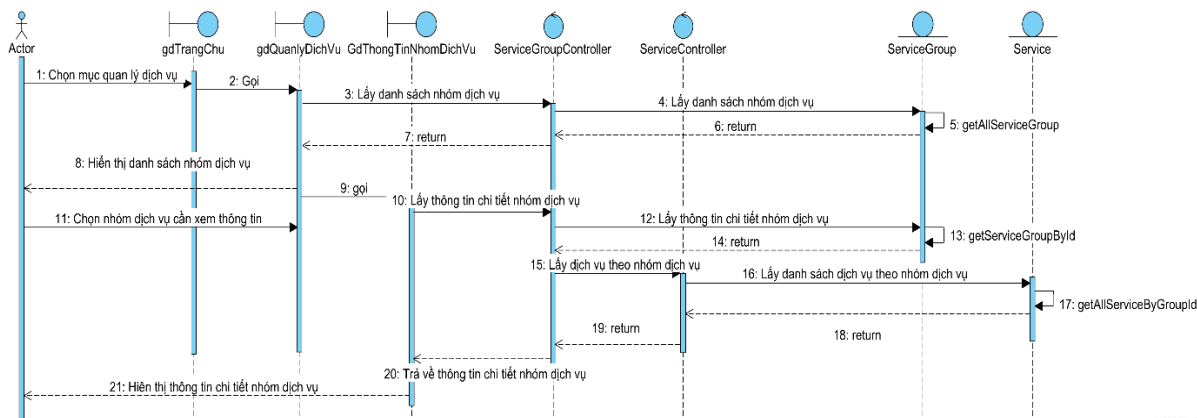
Hình 2.19: Biểu đồ tuần tự chức năng xem chi tiết nhóm dịch vụ
