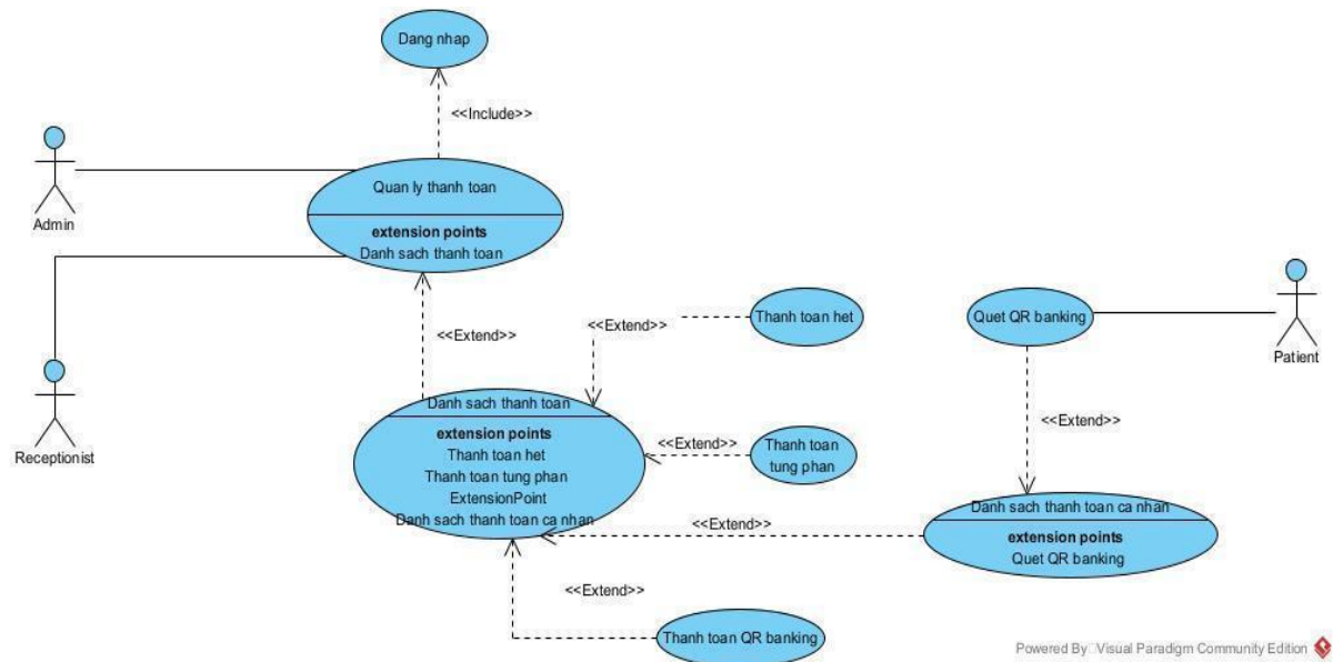
Hình 2.6: Biểu đồ use case chức năng quản lý thanh toán
