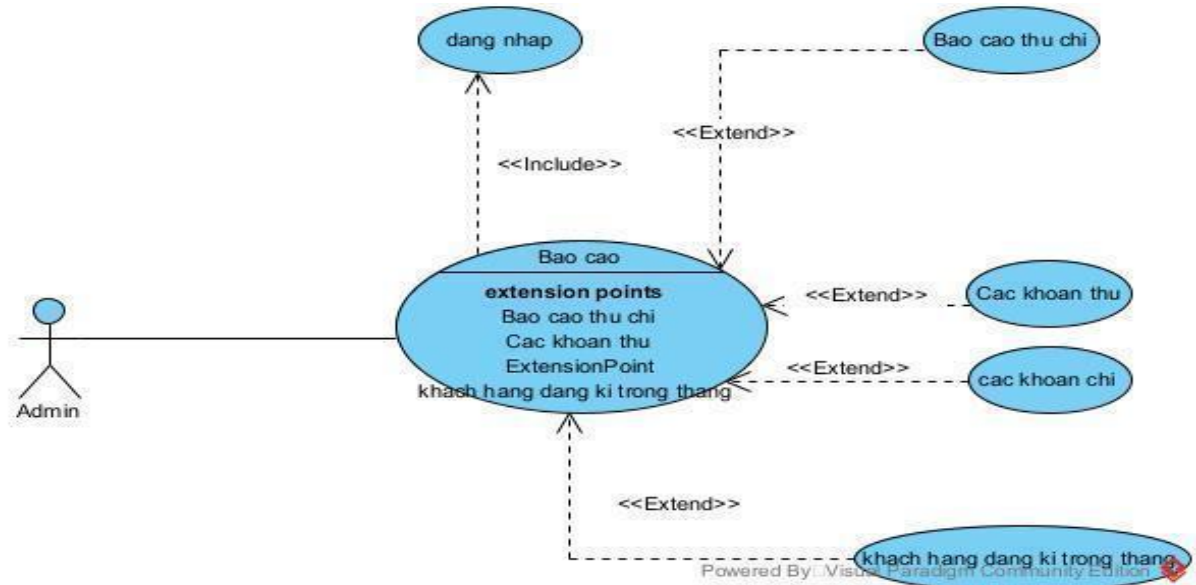
Hình 2.13: Biểu đồ use case chức năng báo cáo
