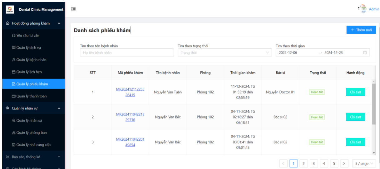
Hình 3.12: Giao diện danh sách phiếu khám
