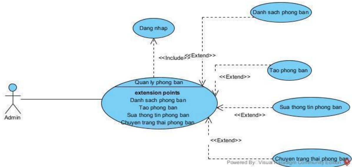
Hình 2.8: Biểu đồ use case chức năng quản lý phòng ban
