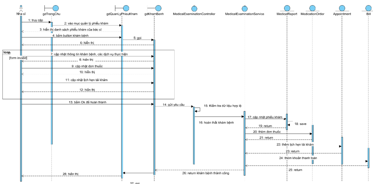
Hình 2.29: Biểu đồ tuần tự chức năng khám bệnh
