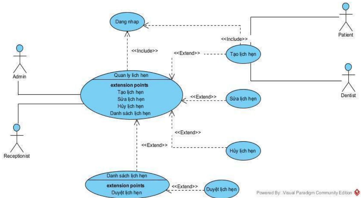
Hình 2.4: Biểu đồ use case chức năng quản lý lịch hẹn
