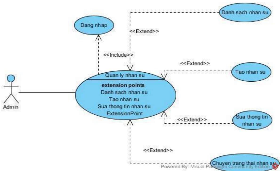
Hình 2.7: Biểu đồ use case chức năng quản lý nhân sự
