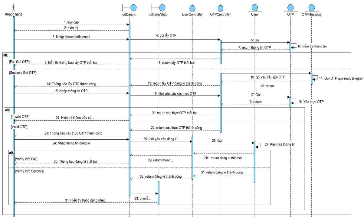
Hình 2.17: Biểu đồ tuần tự chức năng đăng ký
