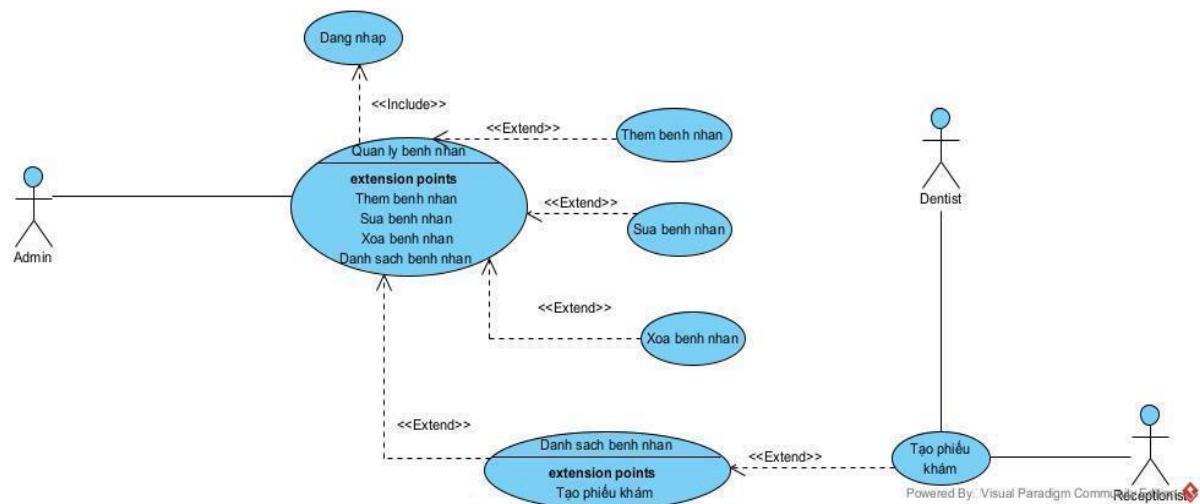
Hình 2.3: Biểu đồ use case chức năng quản lý bệnh nhân
